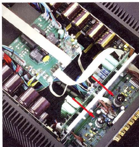
Unico-Kalkül: Die Vorstufen-Röhren (Pfeile) bestimmen den Klang, die Ausgangsverstärker schieben beliebige Ströme nach. Unter der Steuerplatine (links) verstecken sich zwei gigantische Ringkerntrafos.
